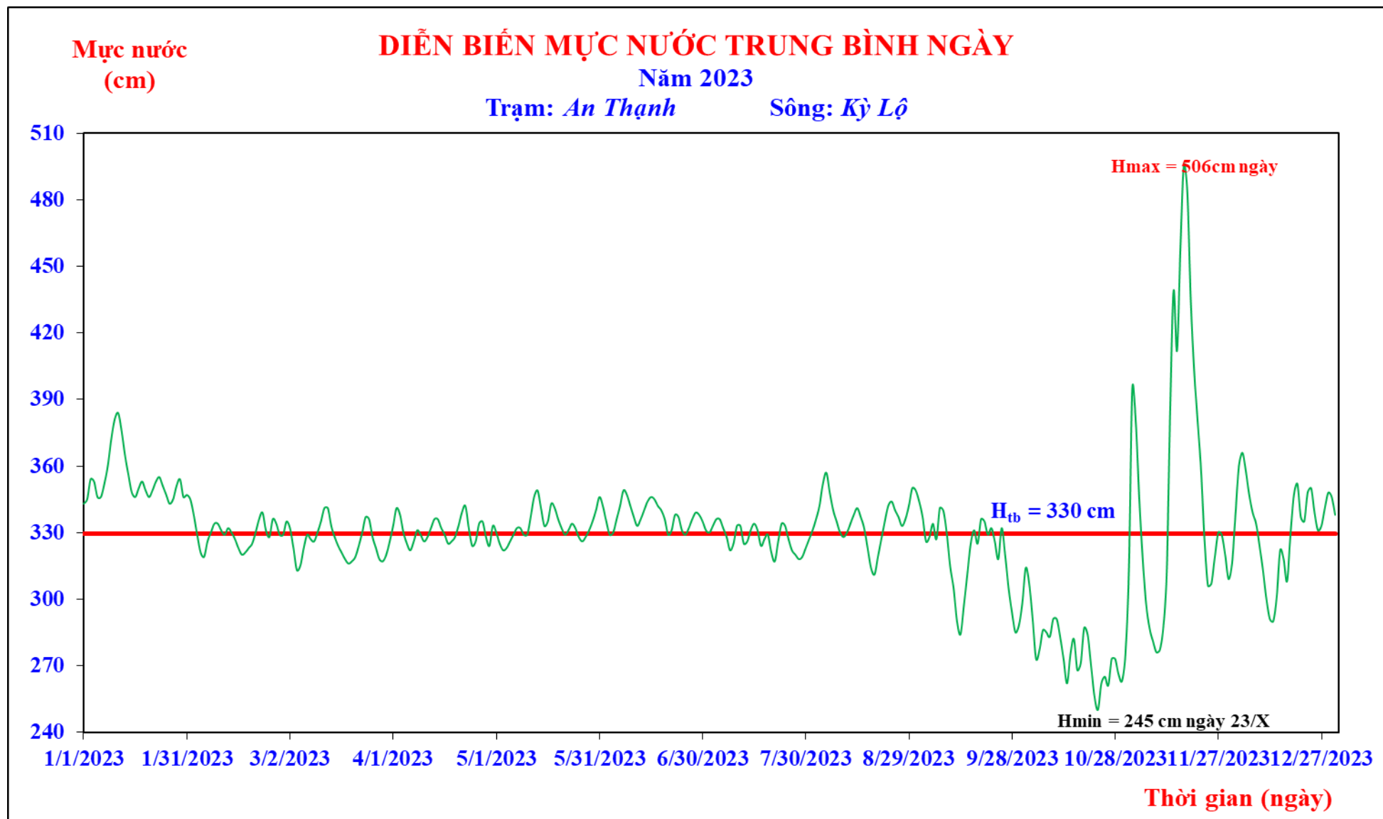
Hình A.2. Diễn biến mực nước trung bình ngày năm 2023 tại trạm An Thạnh
